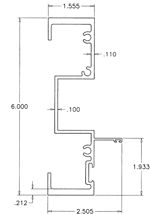
③ FRAME JAMB
